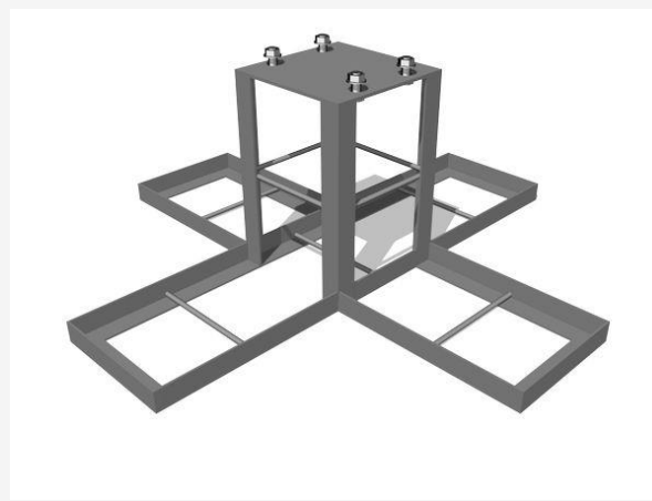
КР013 Закладная карусели
